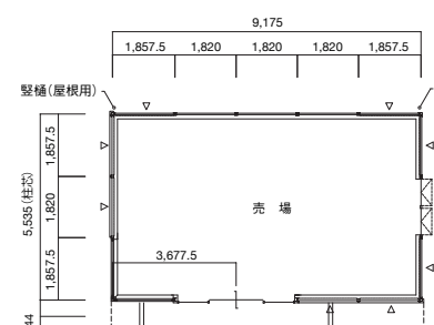
BA2 外壁パネル(鋼製パネルフレームの上 業系サイディングt=15 ヨコ張り)
