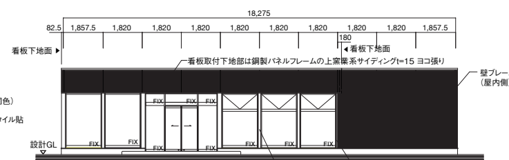
BA2 外壁パネル(鋼製パネルフレームの上 業系サイディングt=16 ヨコ張り)
