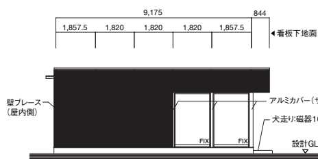
BA2 外壁パネル(鋼製パネルフレームの上 業系サイディングt=16 ヨコ張り)
