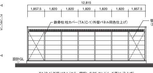
TA(C-1)外壁パネル(カラー鋼板t=0.35 サンドイッチ落し込み式)
