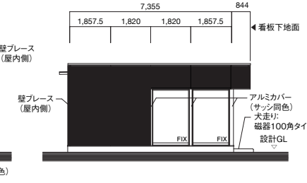
BA2 外壁パネル(鋼製パネルフレームの上 業系サイディングt=16 ヨコ張り)
