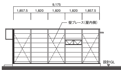
TA(C-1)外壁パネル(カラー鋼板t=0.35 サンドイッチ落し込み式)
