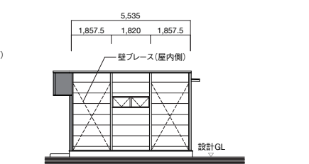
TA(C-1)外壁パネル(カラー鋼板t=0.35 サンドイッチ落し込み式)
