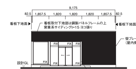
BA2 外壁パネル(鋼製パネルフレームの上 業系サイディングt=15 ヨコ張り)
