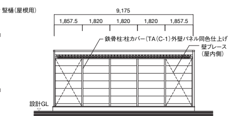
TA(C-1)外壁パネル(カラー鋼板t=0.35 サンドイッチ落し込み式)
