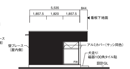
BA2 外壁パネル(鋼製パネルフレームの上 業系サイディングt=15 ヨコ張り)
